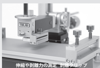
伸縮や剥離力の測定 剥離クリップ
