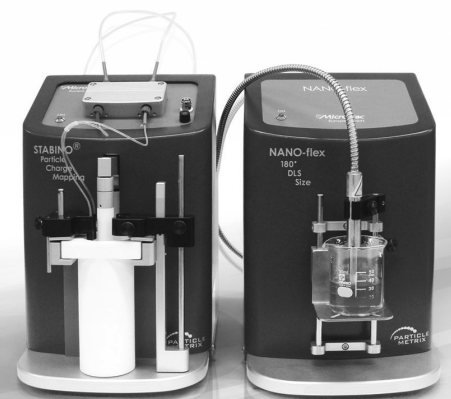
Stabino(左)と NANO-flex(右)との組合せ例
