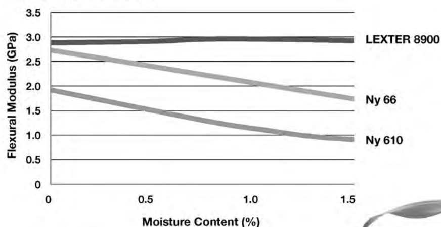
吸水率と弾性率の関係
