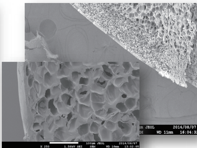
超臨界発泡高分子断面
