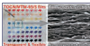
セルロースナノファイバー/モンモリロナイトナノコンポジットフィルムの断面ナノ多層構造
