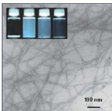
TEMPO触媒酸化によって得られる幅約4ナノメートルのセルロースシングルナノファイバーの電子顕微鏡写真
